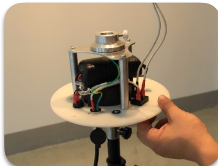
Internal Fan
